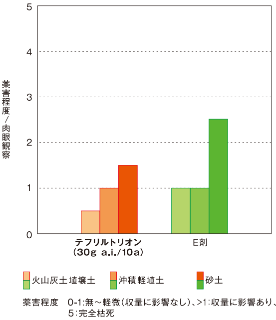
〈テフリルトリオンの土壌別薬害試験〉
